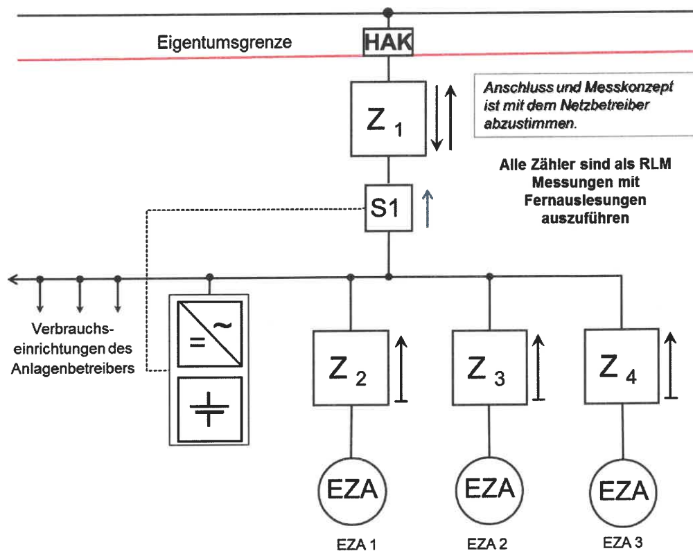
Abbildung 16: Komplexes Anschlussbeispiel mit mehreren EZA und Speicher in der Kundenanlage bei höheren Leistungsgrenzen
