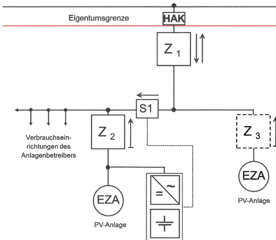
Abbildung 6: Speicher im Erzeugungspfad mit weiterer PV-Anlage
